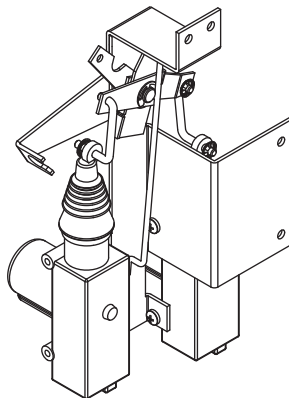
Привод замка M003.500-01
