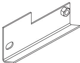
Крышка ручки наружной M002.009
