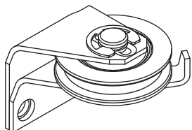
Шкив передний Г012.450-21
