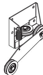
Ролик внутренний M003.430
