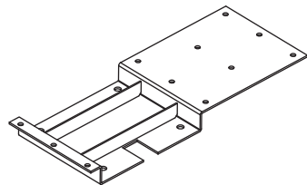
Крышка ручки наружной E001.002
