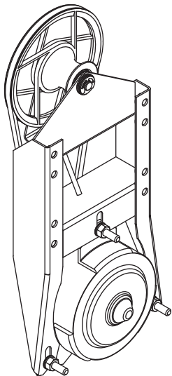
Переключатель верхняя M003.006
