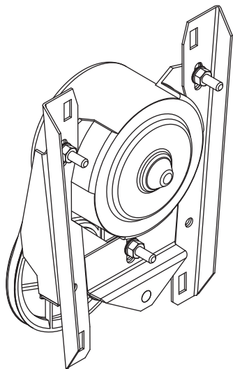
Кронштейн верхний M002.020
