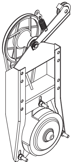
Ролик передний E001.450
