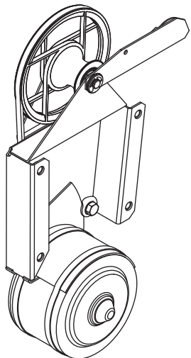
Шкив передний Г012.450-21
