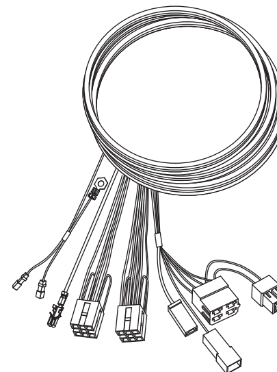
Жгут основной Г012.050 (Баргузин; Соболь)
