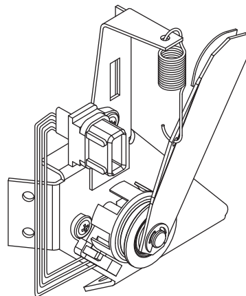
Ролик промежуточный M002.320
