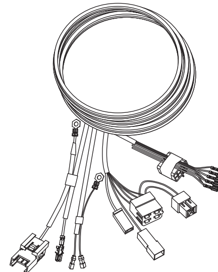
Жгут основной M003.050
